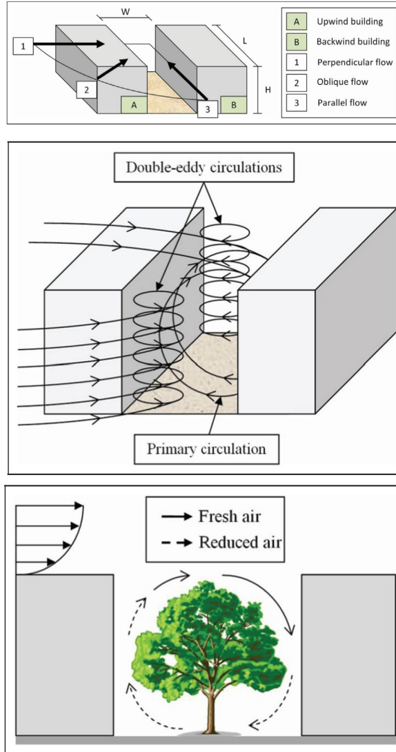
Figura 35. (arriba): Parámetros morfológicos de un cañón urbano. Medio: Generación de turbulencias (movimiento cilíndrico paralelo al suelo) y vórtices (movimiento cilíndrico perpendicular al suelo) con viento perpendicular al cañón. (abajo): Flujo de aire en un cañón arborizado. Fuente: Yazid et al.
